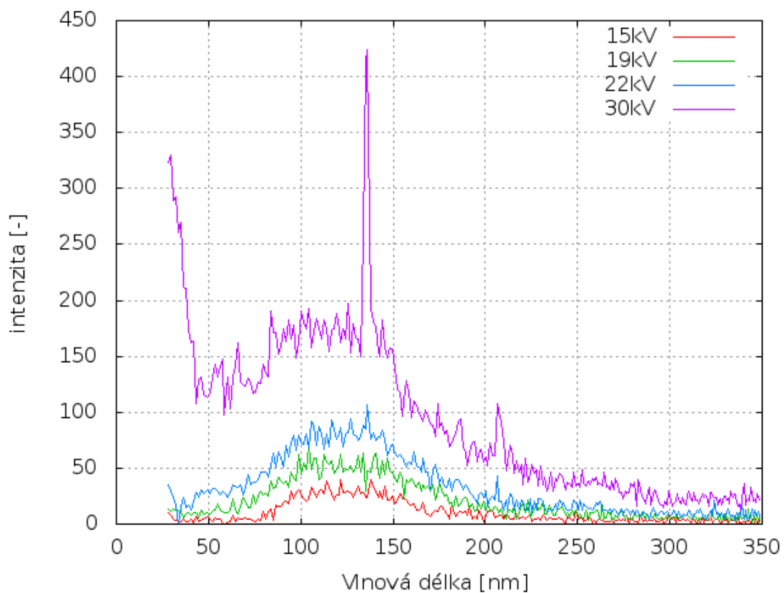
Obrázek 1: Počet detekovaných fotonů za 1s vzhledem k vlnové délce pro Molybdenovou anodu
