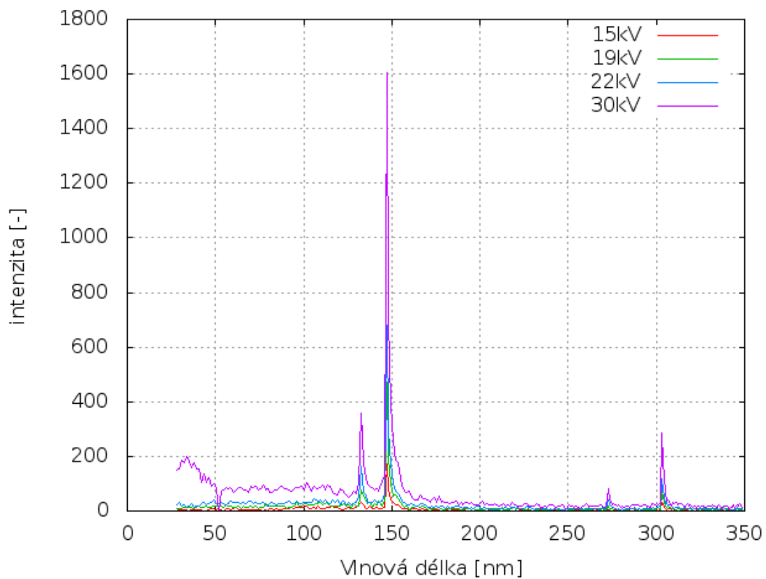
Obrázek 2: Počet detekovaných fotonů za 1s vzhledem k vlnové délce pro Měděnou anodu
