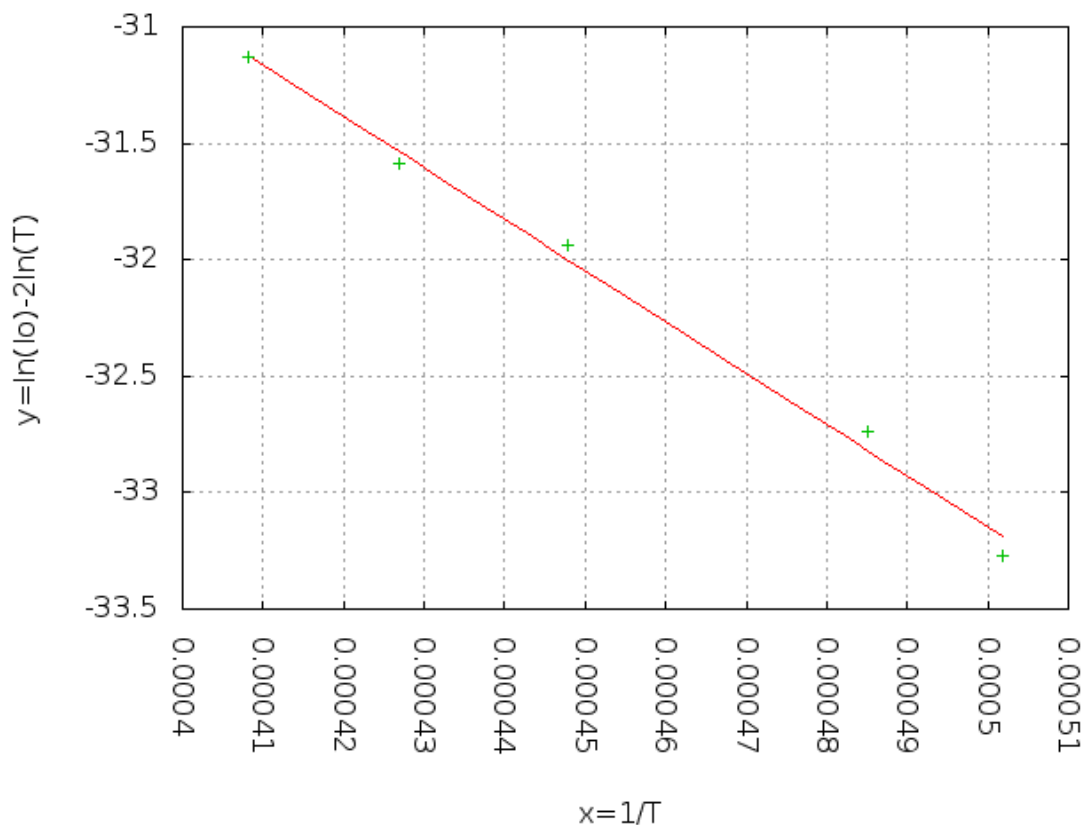
Obrázek 2: Naměřené hodnoty emisního proudu v nasycené oblasti
