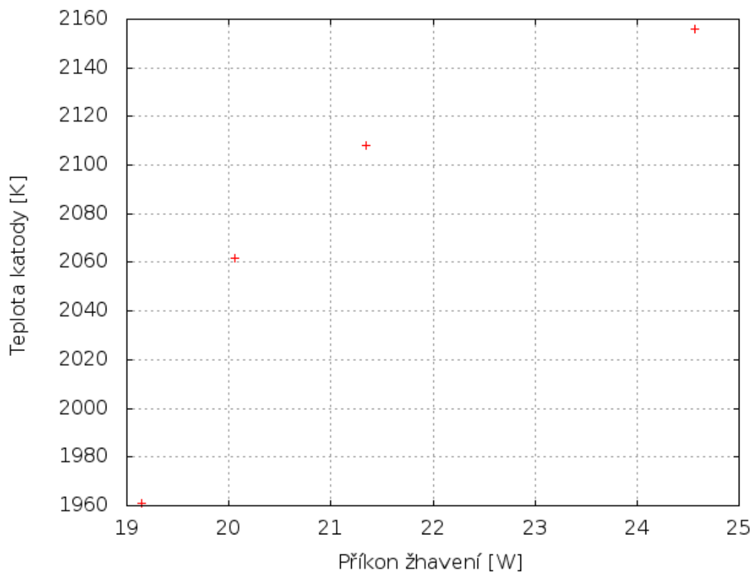
Obrázek 3: Závislost teploty katody na žhavicím příkonu
